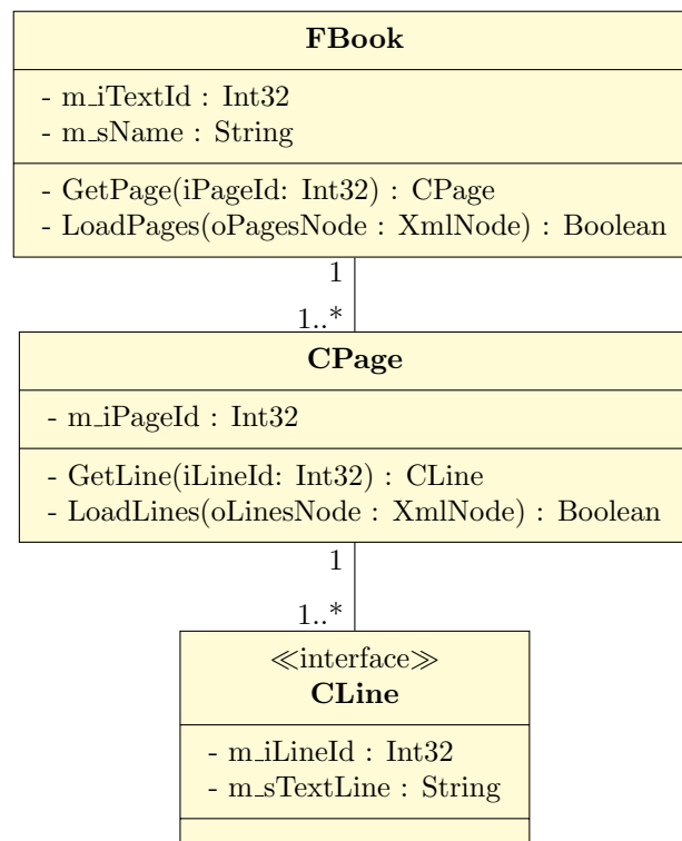
Figura IV.9: Classes de armazenamento da estrutura do texto.
