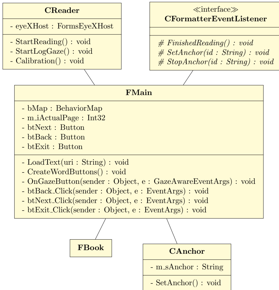
Figura IV.8: Diagrama de classes do leitor.
